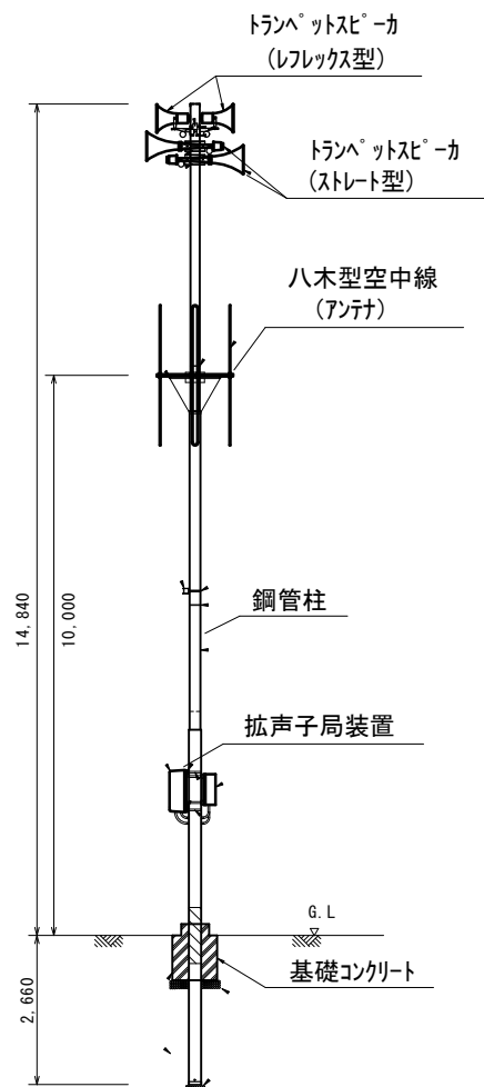
屋外自立局 標準図
